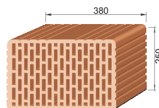
THERMOKRON 38 TK 25 - 18.8 250*380*188
